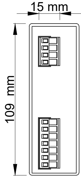
Ön Görünüş
