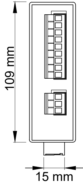
Ön Görünüş
