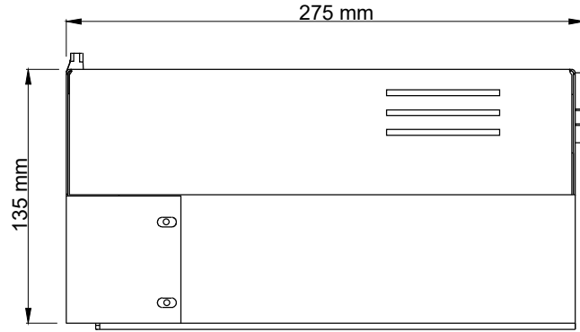
Yan Görünüş
