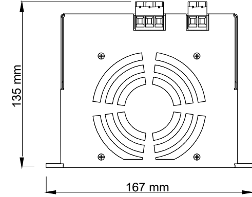
Üst Görünüş
