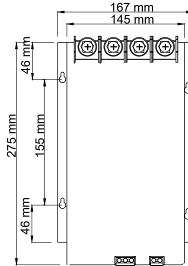
Ön Görünüş
