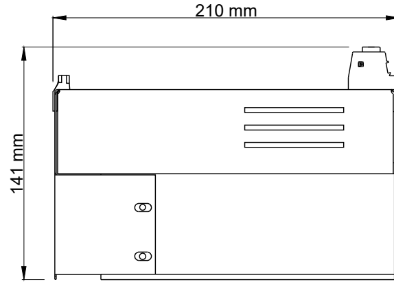
Yan Görünüş
