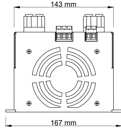
Üst Görünüş
