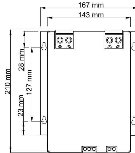
Ön Görünüş
