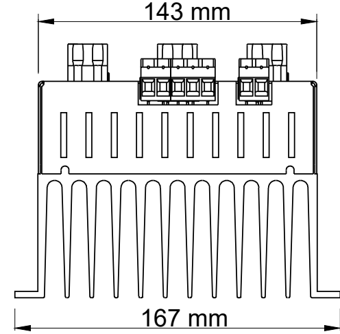
Üst Görünüş
