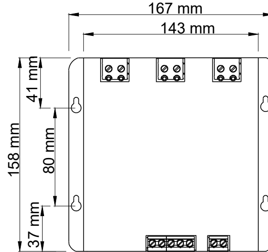
Ön Görünüş
