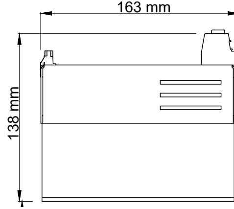
Yan Görünüş
