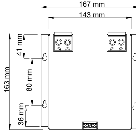
Ön Görünüş
