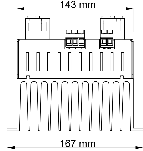
Üst Görünüş
