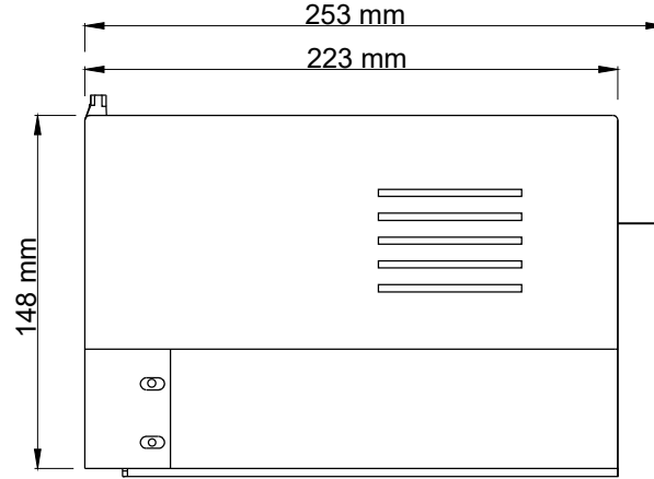
Yan Görünüş
