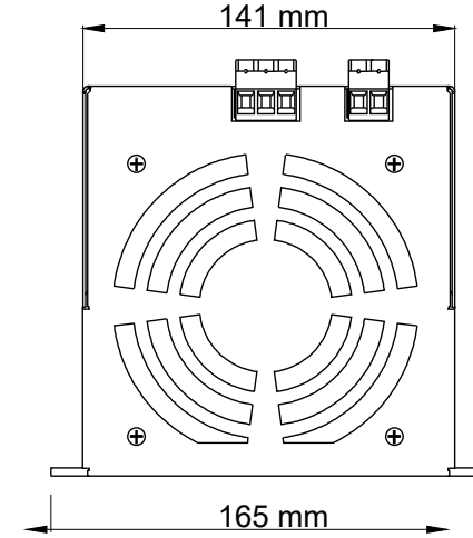
Üst Görünüş
