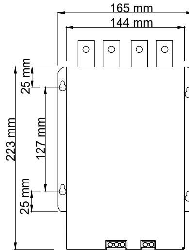
Ön Görünüş
