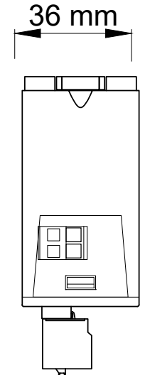
Üst Görünüş
