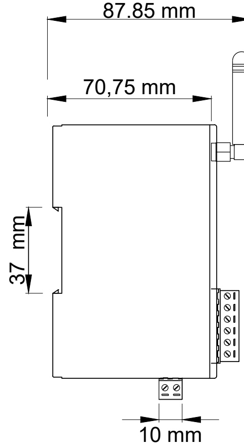
Yan Görünüş
