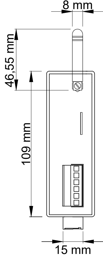
Ön Görünüş
