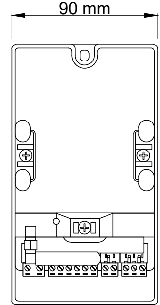
Ön Görünüş
