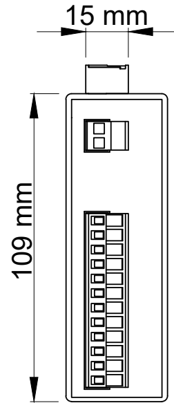
Ön Görünüş
