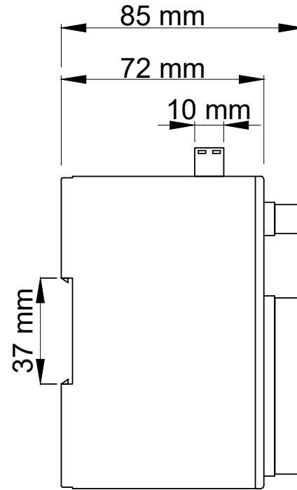
Yan Görünüş
