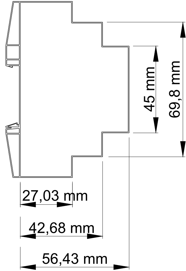
Yan Görünüş
