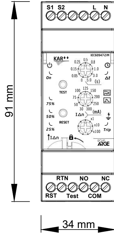
ÖN GÖRÜNÜM
