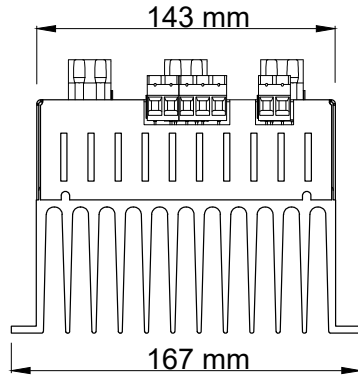
Üst Görünüş
