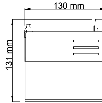
Yan Görünüş
