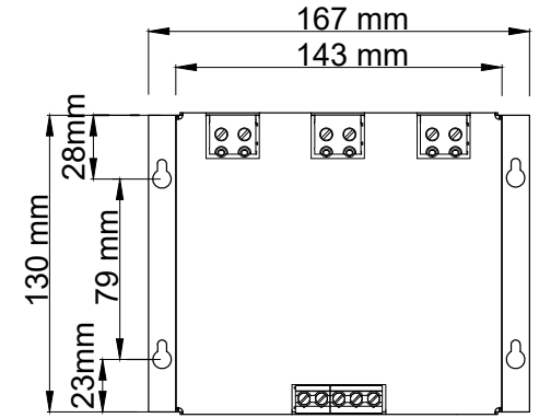
Ön Görünüş
