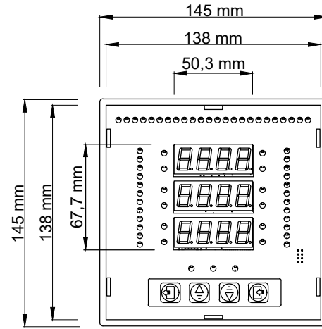
Ön Görünüş
