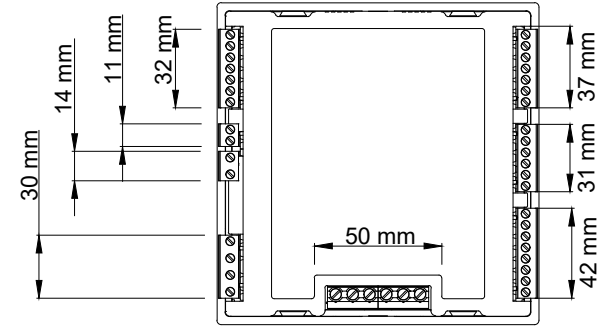
Arka Görünüş
