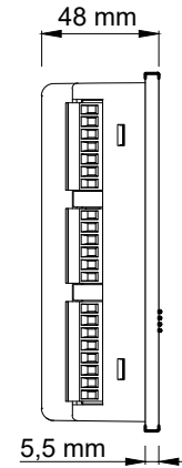
Yan Görünüş
