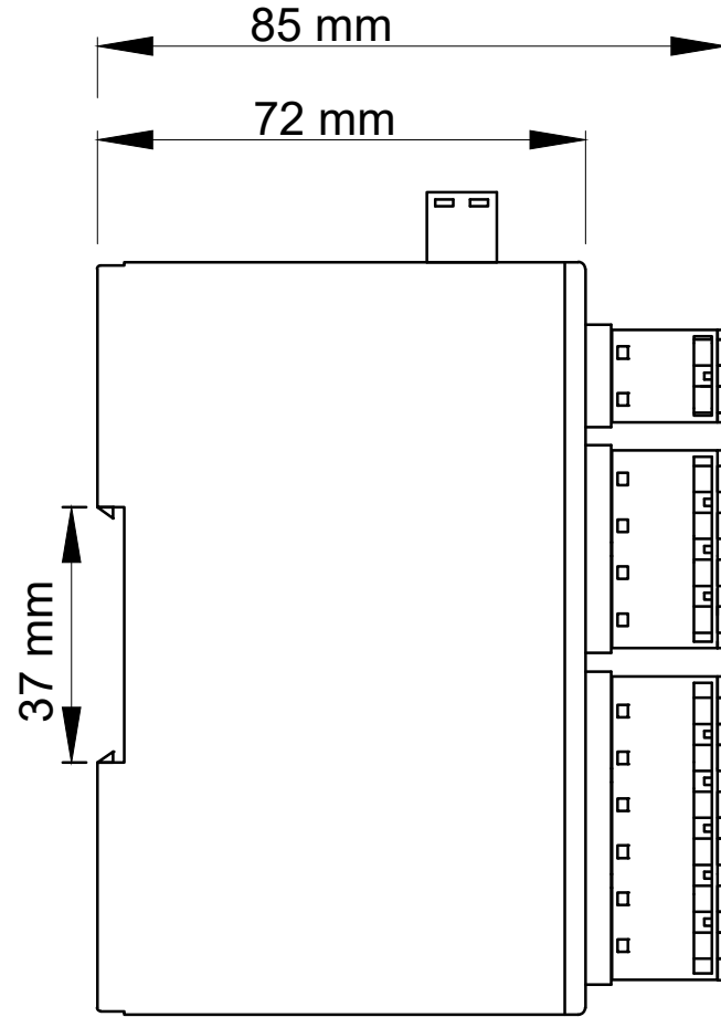
Yan Görünüş
