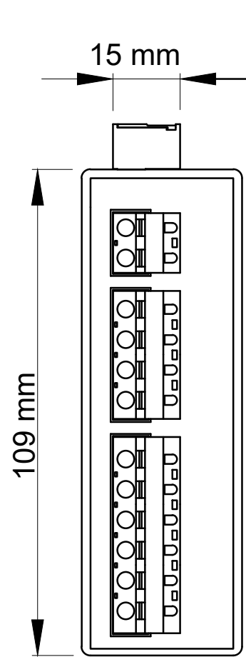
Ön Görünüş
