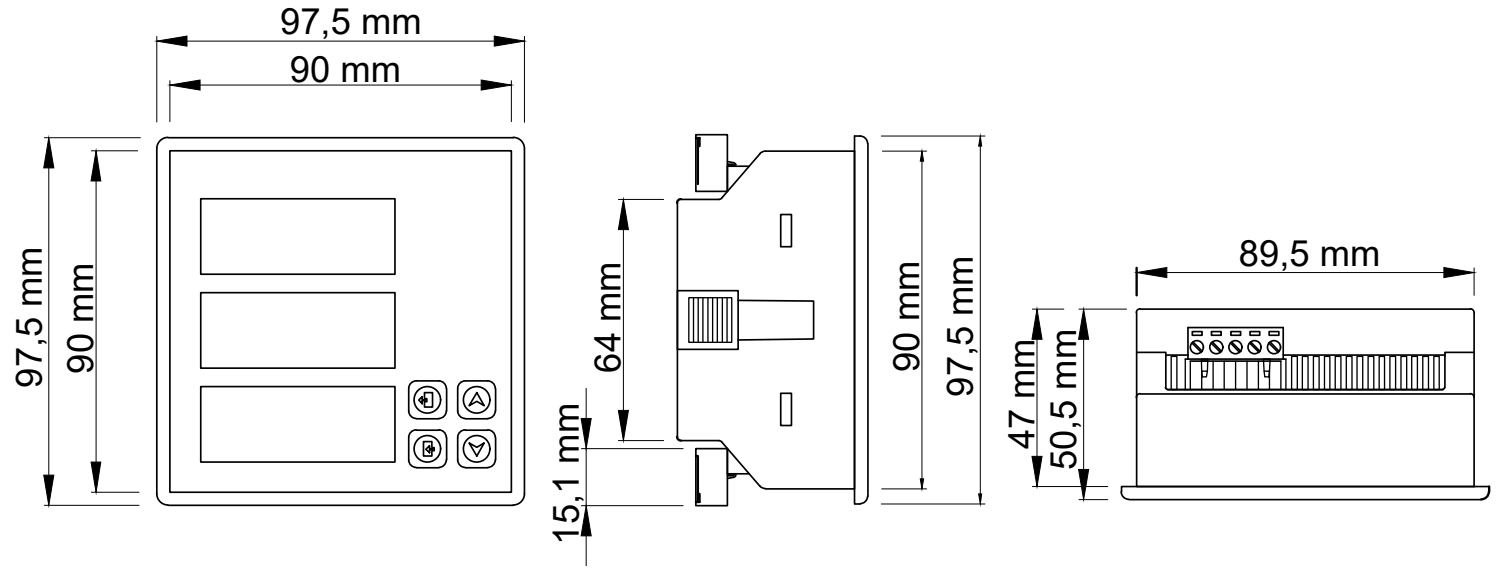
Ön Görünüş
