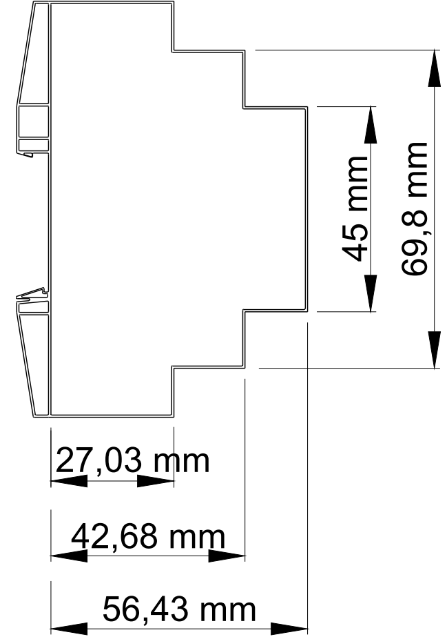
Yan Görünüş
