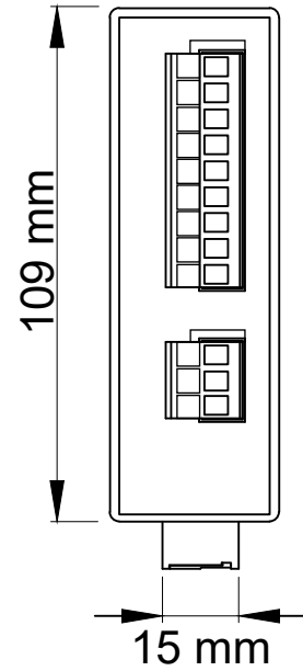
Ön Görünüş
