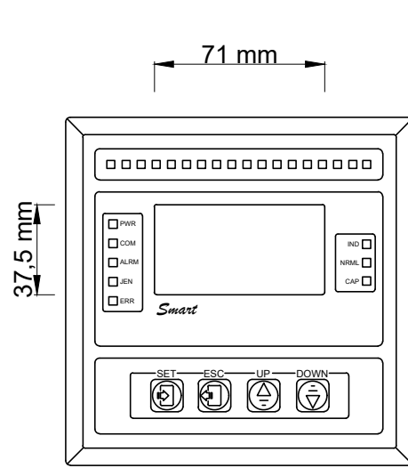
Ön Görünüş
