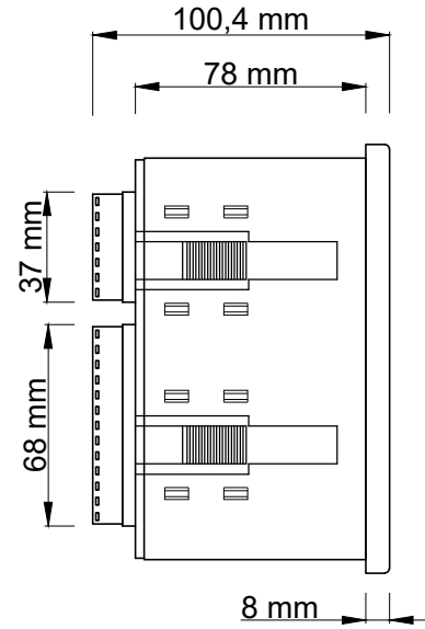
Yan Görünüş
