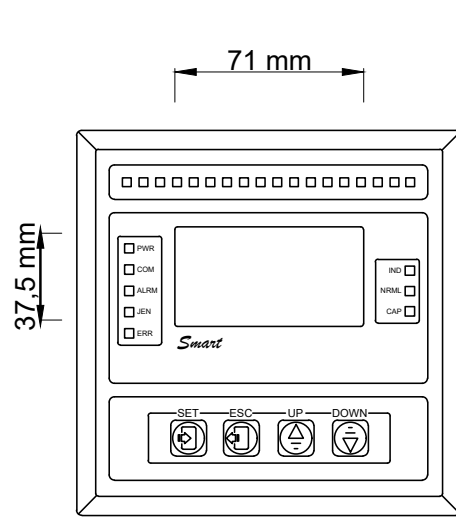
Ön Görünüş
