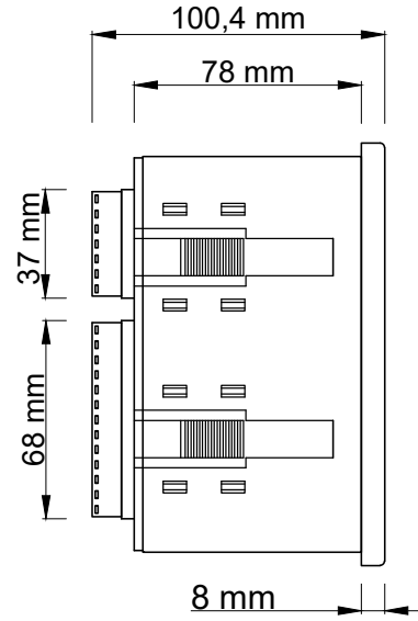
Yan Görünüş
