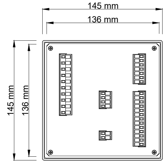
Arka Görünüş
