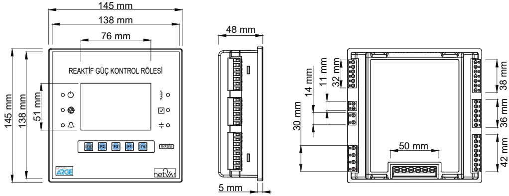
RKRS 07/12/18 SVC'li Reaktif Güç Kontrol Rölesi
