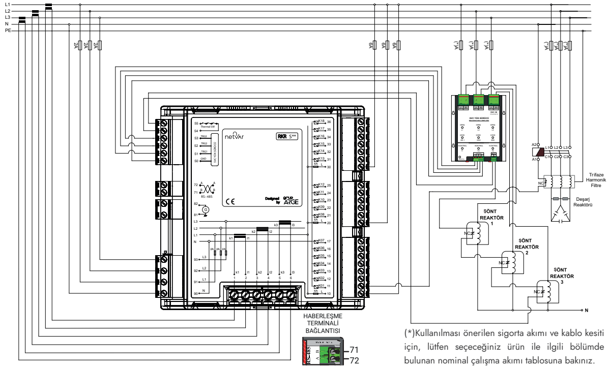
RKRS 07/12/18 SVC'li Reaktif Güç Kontrol Rölesi
