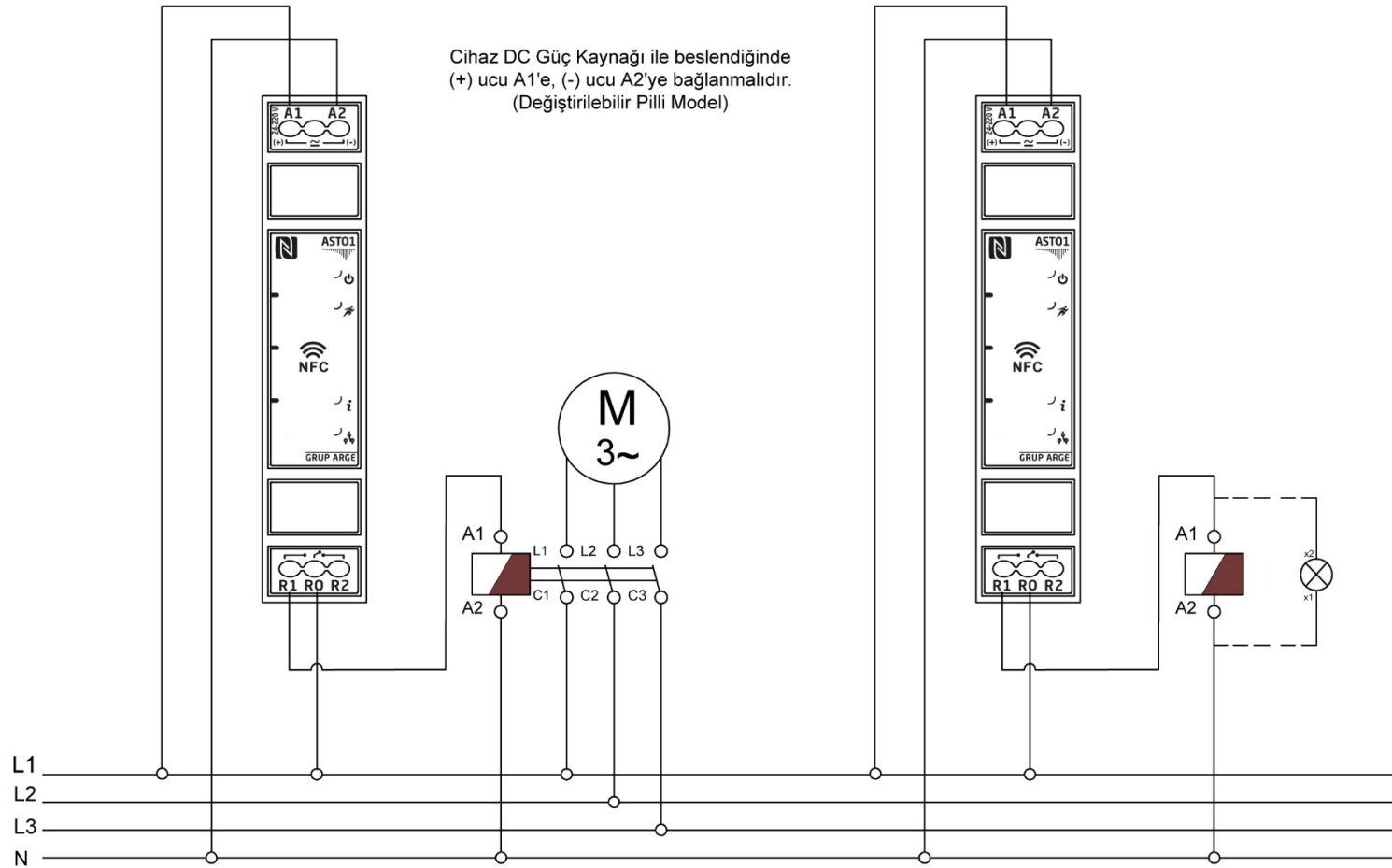
Bağlantı Şeması
