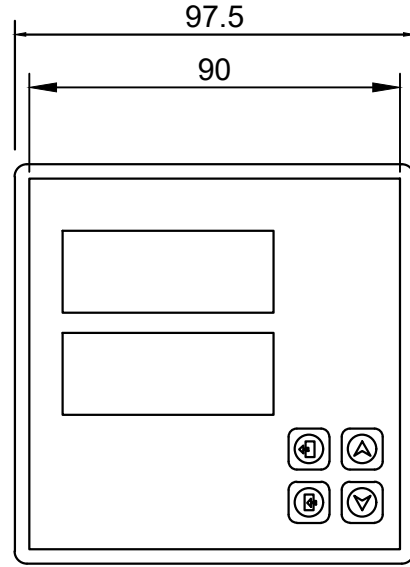
ÖN GÖRÜNÜŞ
