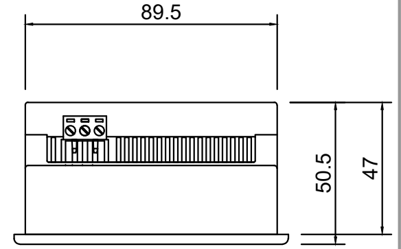
ÜST GÖRÜNÜŞ
