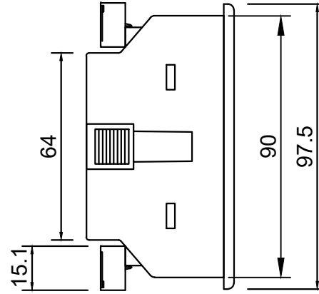
YAN GÖRÜNÜŞ
