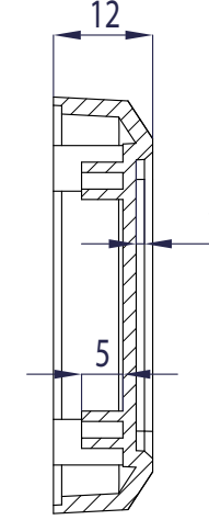
KESİT A-A
