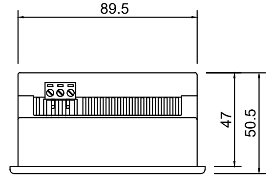
ÜST GÖRÜNÜŞ
