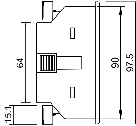
YAN GÖRÜNÜŞ
