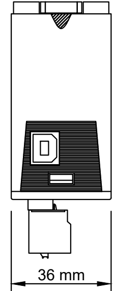
ÜST GÖRÜNÜŞ
