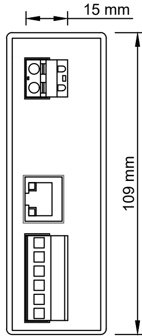
ÖN GÖRÜNÜŞ
