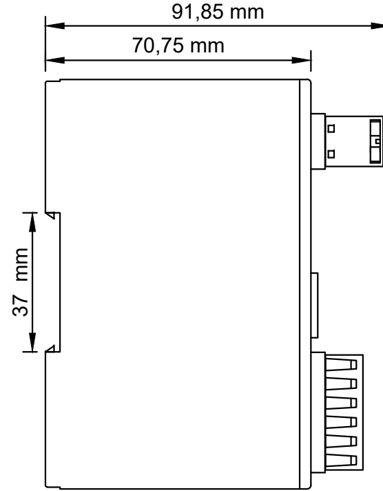
YAN GÖRÜNÜŞ
