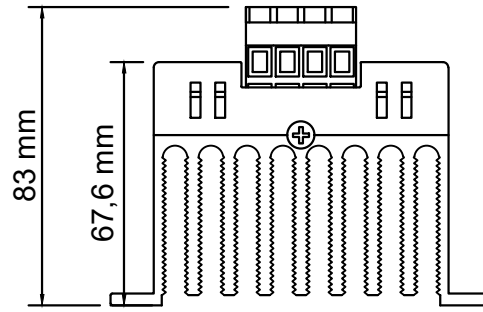
ÖN GÖRÜNÜŞ
