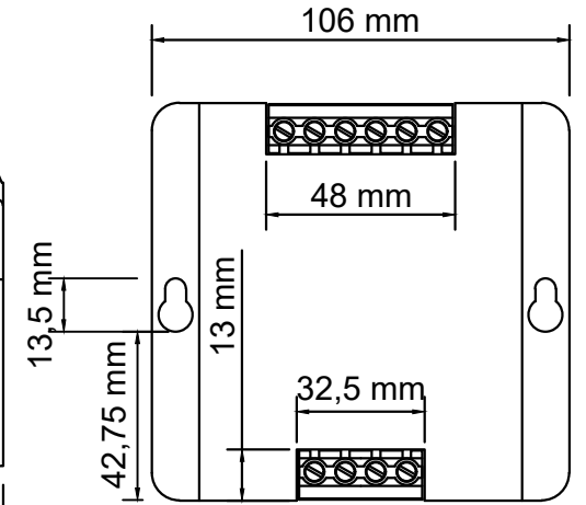
ÜST GÖRÜNÜŞ
