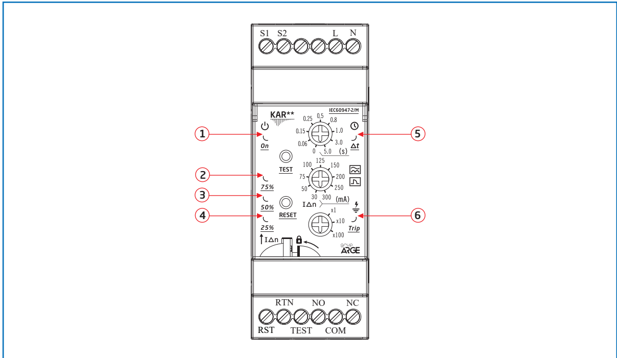
Şekil 3: KAR01-KAR11 Kaçak Akım Rölesi Ön Görünümü
