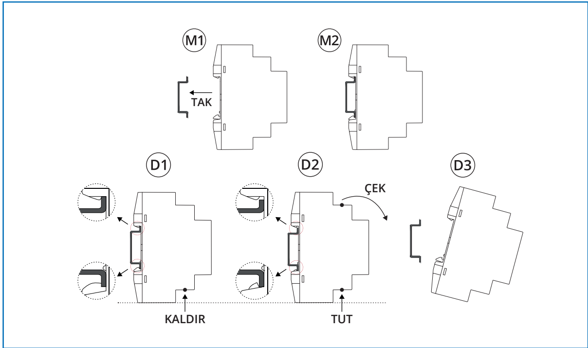
Şekil 2 : KAR01-KAR11 Kaçak Akım Rölesi Ürün Montajı ve Demontajı
