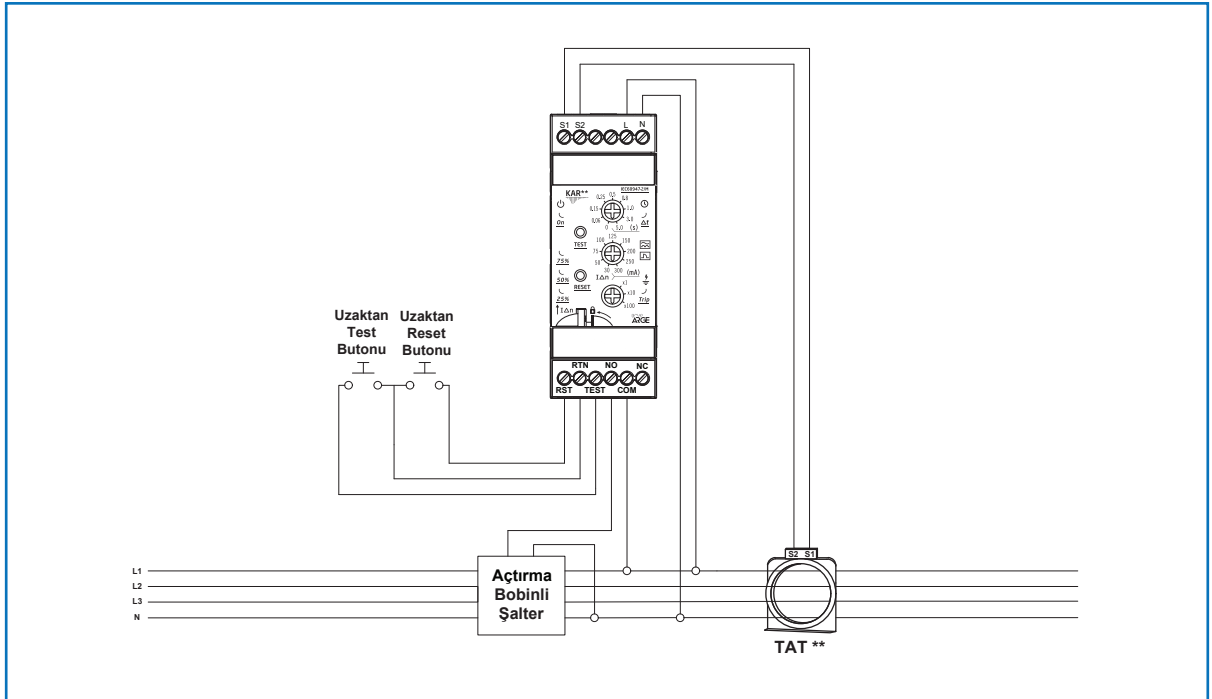
Şekil 4: Toroidal Kaçak Akım Rölesi Bağlantı Şeması
