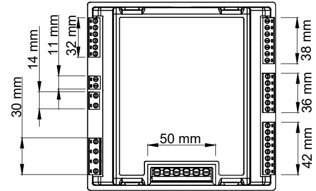
Arka Görünüş
